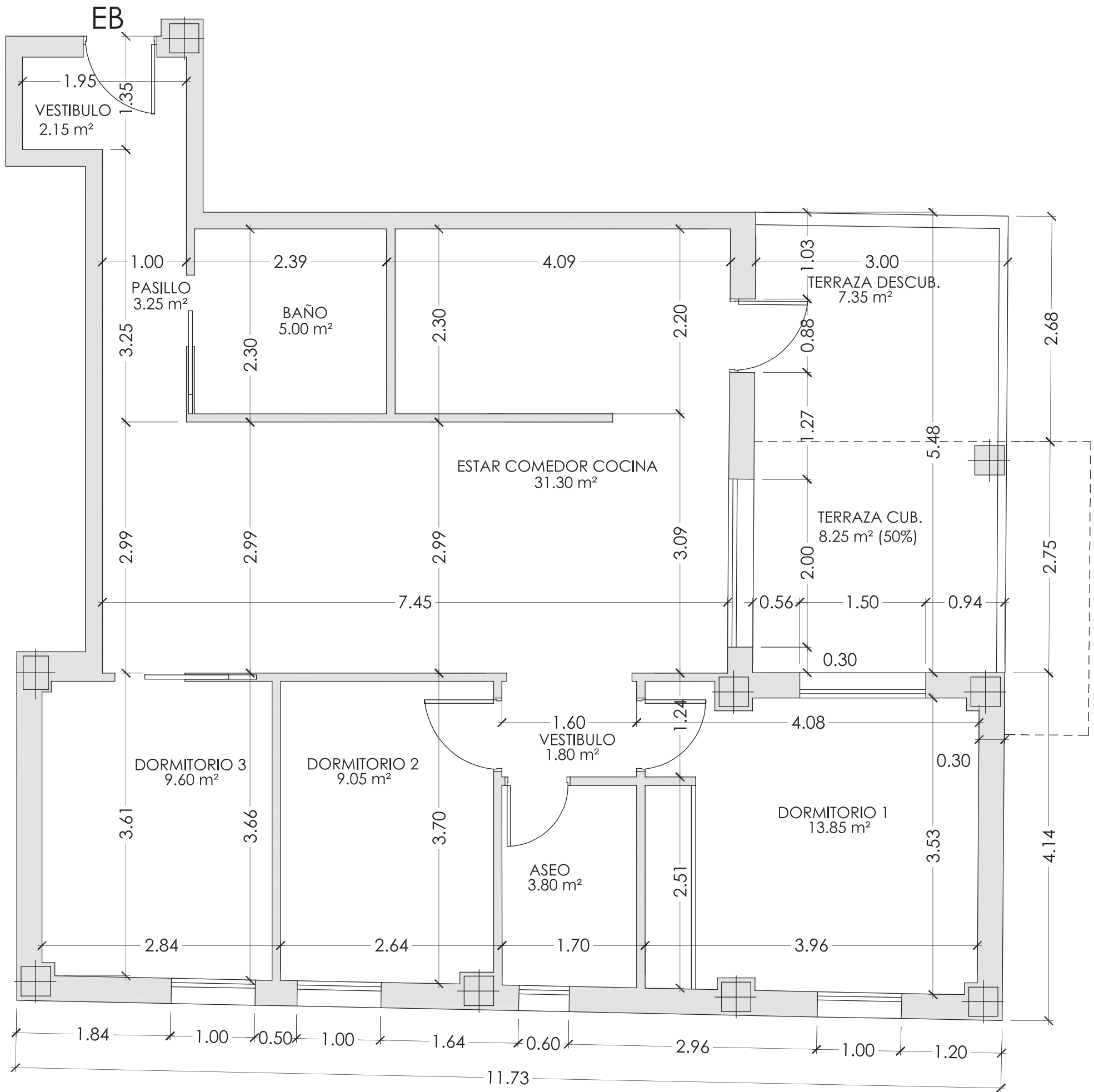
EDIFICIO REAL- ARMILLA. Entreplanta B (Cotas)
